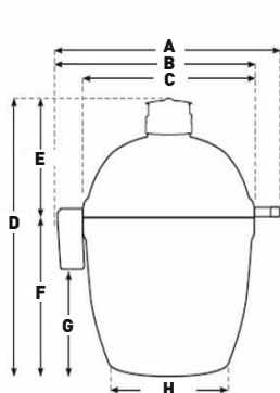
ZIJAAZICHT
