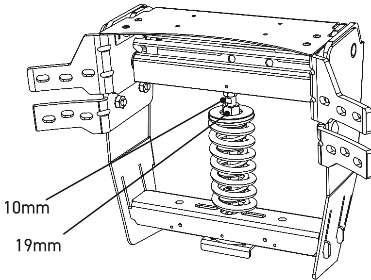
ALTERNATIEF SCHARNIER
