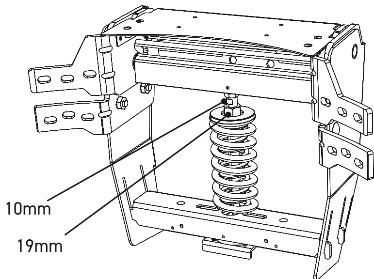
ALTERNATIV HINGE
